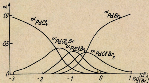
3. ábra. A vegyes ligandum komplexek móltörtje, mint a két ligandum koncentrációja hányadosának függvénye a \text{Pd}^{2+}-\text{Cl}^--\text{Br}^- rendszerben [12]
