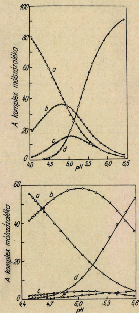
4. ábra. A különböző komplexek eloszlása a pH függvényében a \text{Cu}^{2+}-2,7\text{-diamino-szuberinsav (DAS)} rendszerben
