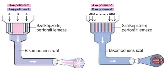
6. ábra. Példák a bikomponens szálképzésre
